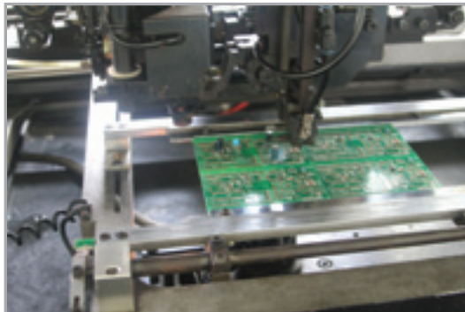
Pose automatique des composants axiaux et radiaux.
