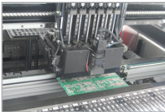
Pose automatique des composants CMS.
