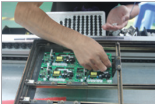
Insertion manuelle des composants volumineux.
