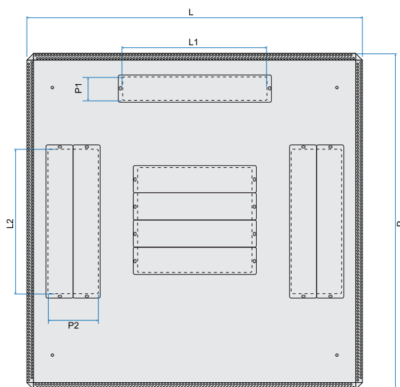
Exemple de capot pour baie ligne 500 largeur 800.
