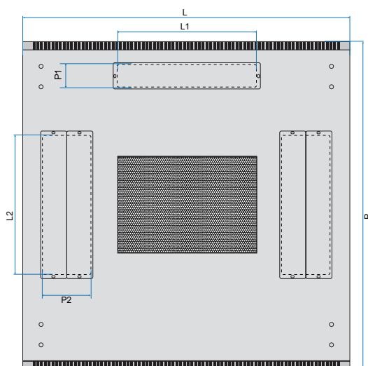
Exemple de capot pour baie ligne 800 largeur 800.
