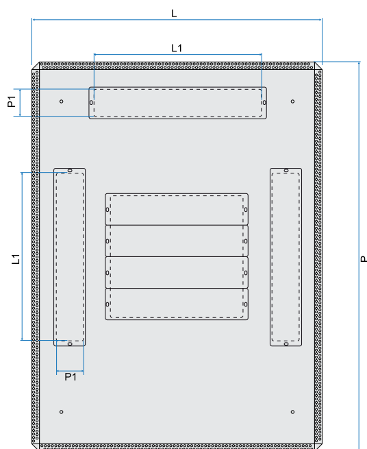
Exemple de capot pour baie ligne 500 largeur 600.
