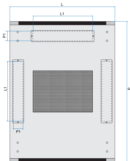
Exemple de capot pour baie ligne 800 largeur 600.
