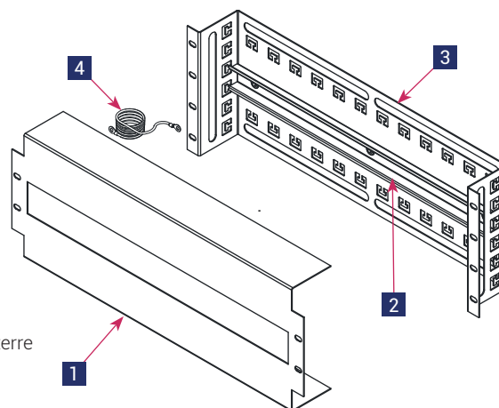
vue éclatée.
