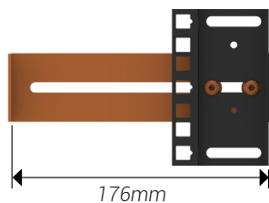
vue avec équerres de racking réglées en retrait
