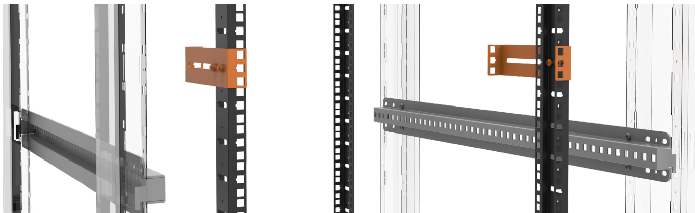
vue avec équerres de racking réglées en retrait
